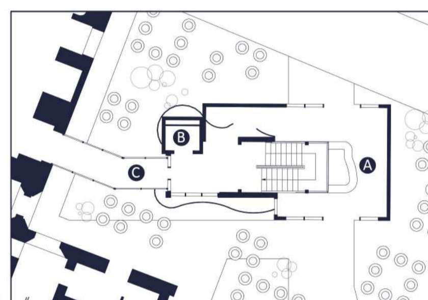
PIANTA PIANO TERRA: A- Ingresso/caffetteria, 25 mq B- Ascensore e cavedio impiantistico C- Connessione con ambienti museo
